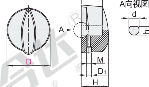
内螺纹型 HAQ17
