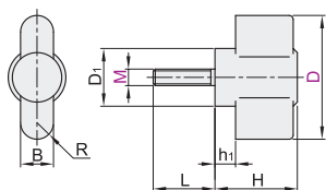
外螺纹型 HAQ11
