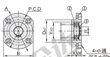
单件·支持侧 LHF04
