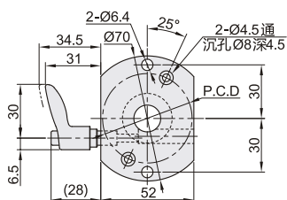
单件·防转动固定件(适用大型数字式位置显示器) LHF10
