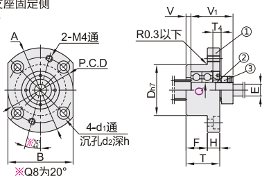
单件·防转动固定件 LHF08
