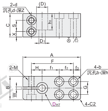
偏置型 RCG21/22
