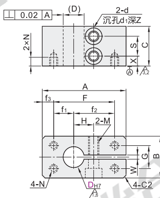
螺孔型 RCG11/12
