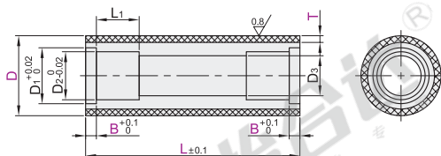
单向对称型 QAA31/32
