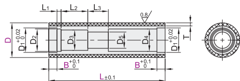
单向薄壁型 QAA26/27
