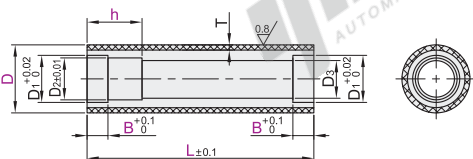
单向标准型 QAA21/22
