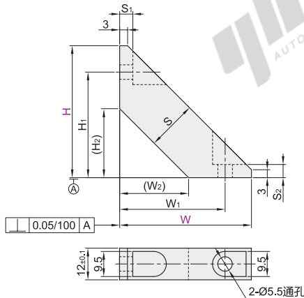
沉孔型 ZGC11/12/13/14
