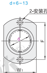
对边法兰型 LMQ21/22
