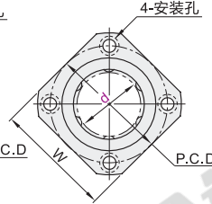
方法兰型 LMQ11/12
