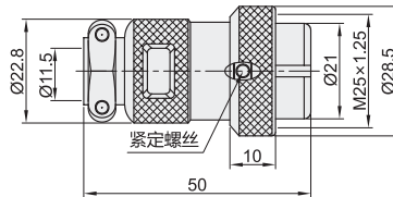
规格: 40
