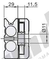
截面B-B
