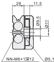
截面A-A
