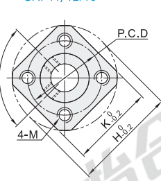
方法兰型 GAF11/12/16
