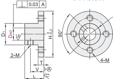
圆法兰型 GAF01/02/06
