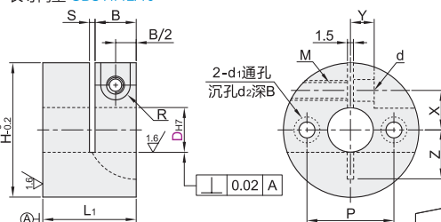
长导向型 GBS11/12/16
