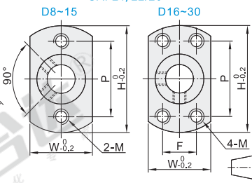
对边法兰型 GAF21/22/26
