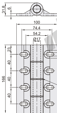
横向腰孔型 HFC88
