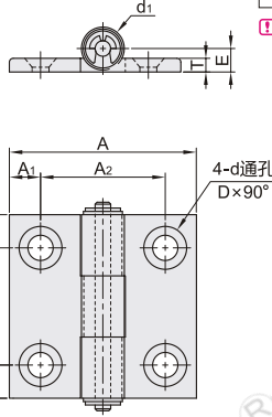
锥孔型 E-HFC89 E-HFC90
