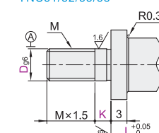
带肩型-外螺纹型 YNC51/52/55/58
