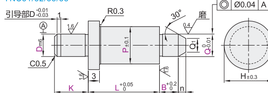
带肩型-标准型 YNC31/32/35/38
