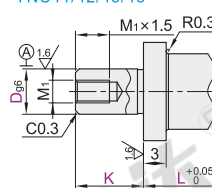
带肩型-内螺纹型 YNC41/42/45/48
