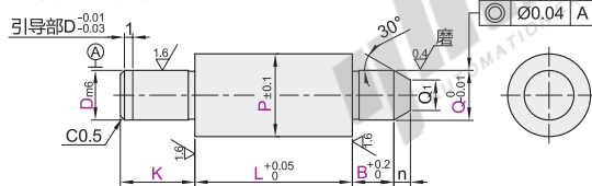
无肩型-标准型 YNC01/02/05/08
