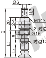
弹簧式顶部真空端口 J-WEU06
