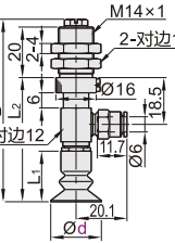
弹簧式侧面真空端口 J-WEU11
