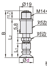
弹簧式直接安装型 J-WEU16
