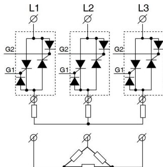
K3 三相三线全控功率模块星型、 三角型接线图（单相可控硅反并联）
