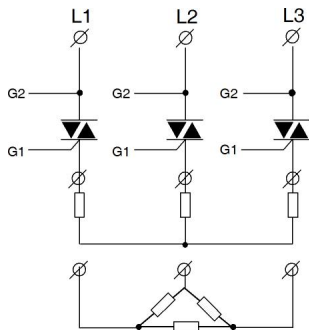
K3 三相三线星型、 三角型接线图（双向可控硅）
