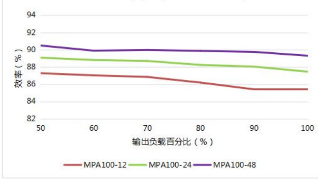
效率Vs输出负载 ( Vin=115VAC )
