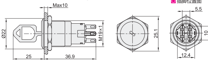
插脚位置图
