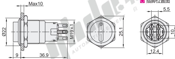
插脚位置图
