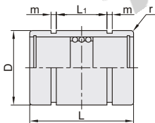
单衬型 LNC01
