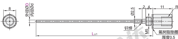
外螺纹短型-软管接头型 NHR37
