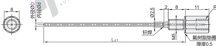
外螺纹长型-内螺纹 NHR24
