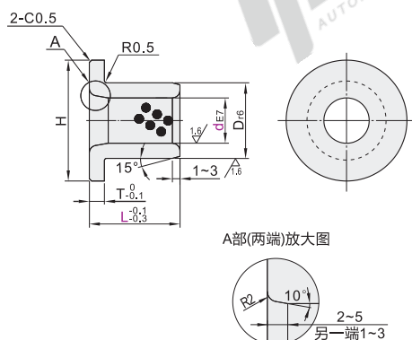
标准型 OFN01
