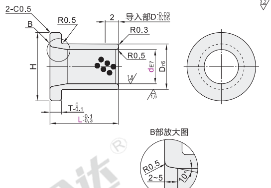
薄壁型 OFN02
