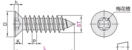
梅花槽沉头自攻螺钉 TBS65
