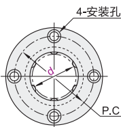
圆法兰型 Y-GVC31/32
