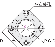
方法兰型 Y-GVC41/42
