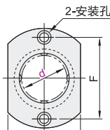
对边法兰型 Y-GVC51/52
