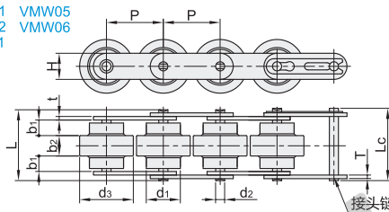
接头链接
