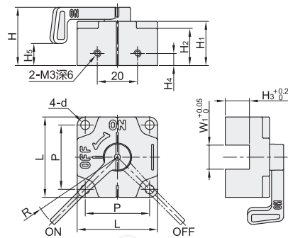
手柄型 HCB04
