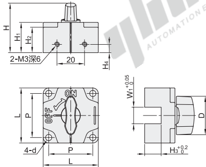
旋钮型 HCB01/02/03
