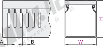
□ W≤70mm线槽底部孔尺寸
