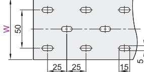
□ W≥80mm线槽底部孔尺寸
