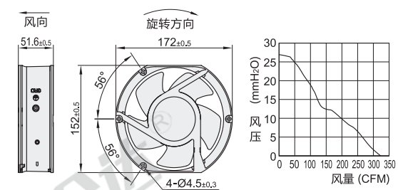
外形尺寸: 172
