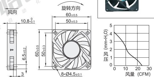
外形尺寸: 6010
