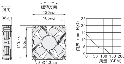
外形尺寸: 120/120A12
