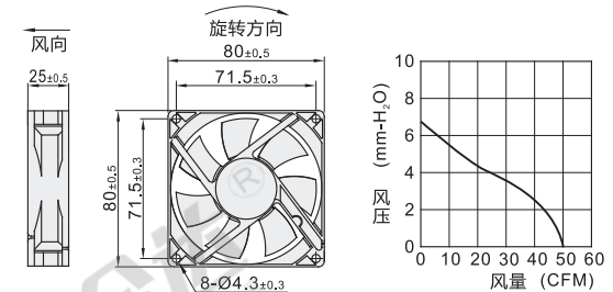
外形尺寸: 80/80B12/80B48
