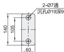
键盘托盘尺寸
