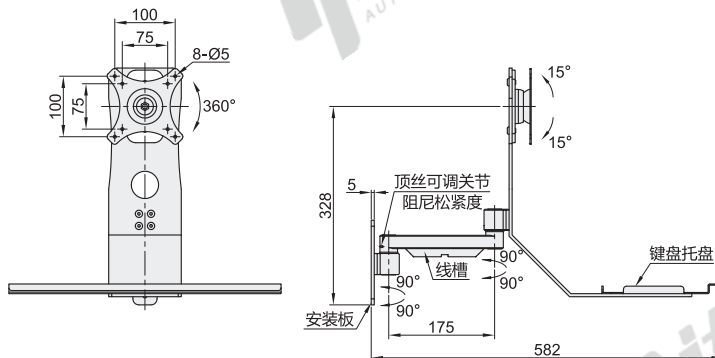
键盘不可折叠 E-NHL50
