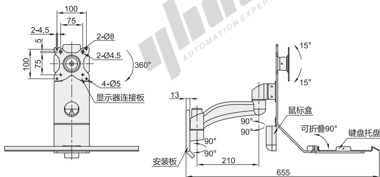
键盘可折叠 NHL52
