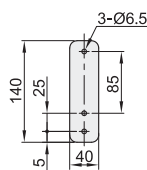
安装板尺寸
