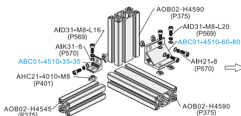
分解图
