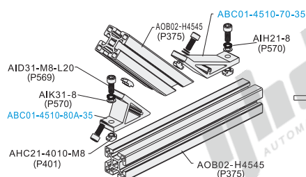
分解图
