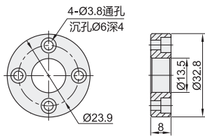
B1(闭口磁环)
