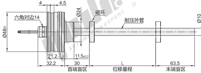
B1(闭口磁环)
