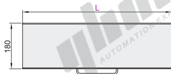
键盘托盘尺寸
