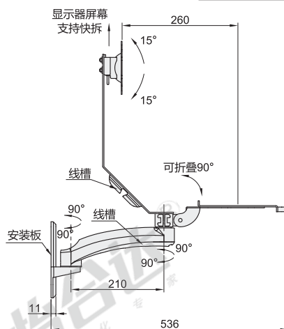
安装板尺寸
