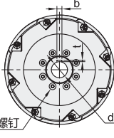
左轮 CNG85
