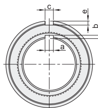
CSK...PP(带内外键槽)
