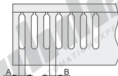
W < 80mm线槽底部孔尺寸
