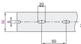
W < 80mm线槽底部孔尺寸
