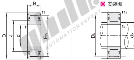
安装图
