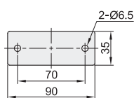
■ 安装板尺寸
