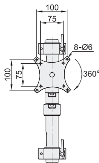
双臂 NHD99
