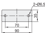
■ 安装板尺寸
