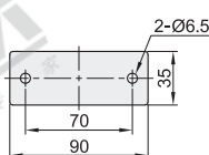
■ 安装板尺寸
