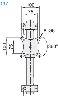
无臂 NHD97
