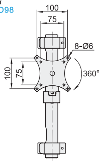
单臂 NHD98
