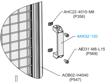
分解图
