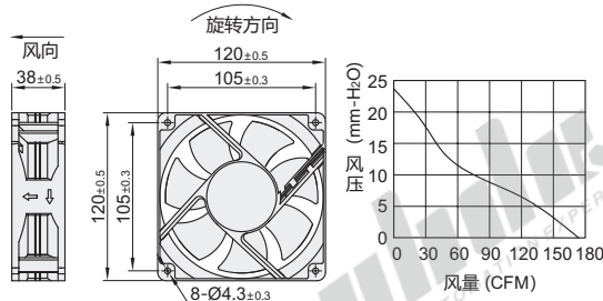
外形尺寸: 12038
