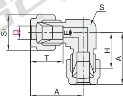
等径·弯接头
