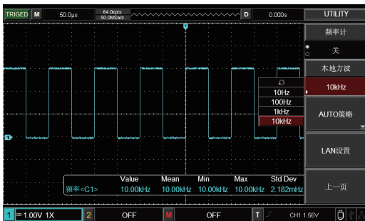
多种频率输出标准方波可选
