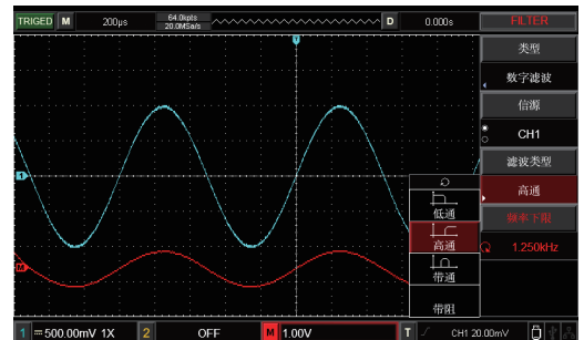
丰富的Math功能: 数学运算, FFT, 数字滤波
