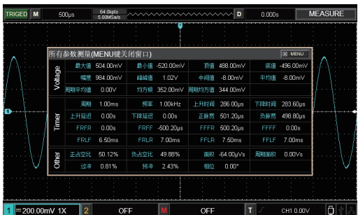
多种波形参数自动测量
