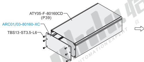
分解图
