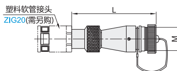
ZD(直式对接塑料软管插座)
