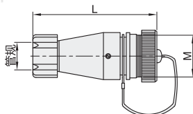
ZP(直式对接金属软管插座)
