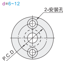
圆法兰型 E-OCR01
