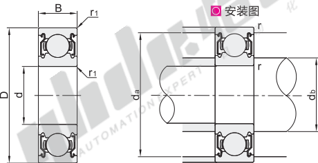
安装图
