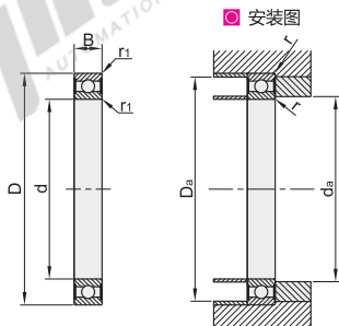
安装图
