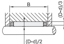
安装图2
