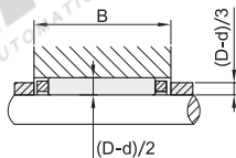
安装图1
