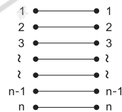
内部接线
