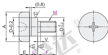
十字槽型 MJT61/62/66
