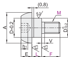
圆头螺钉型 MJT41/42/46
