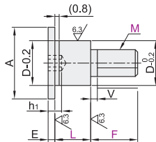
超短头型 MJT01/02/06
