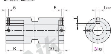
键槽+螺孔型
