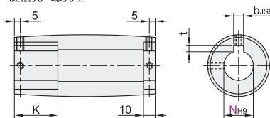
键槽+螺孔型
