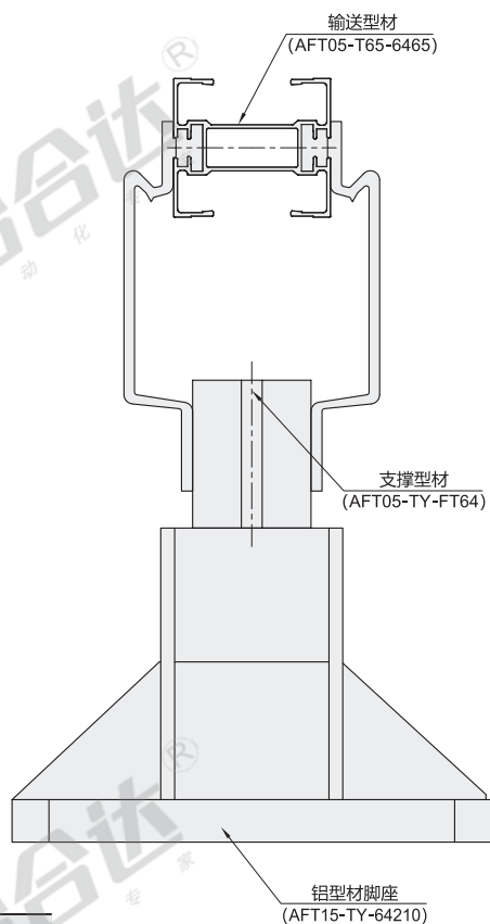
支腿装配示意图
