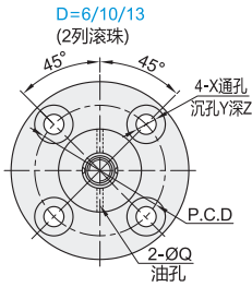
A向视图
