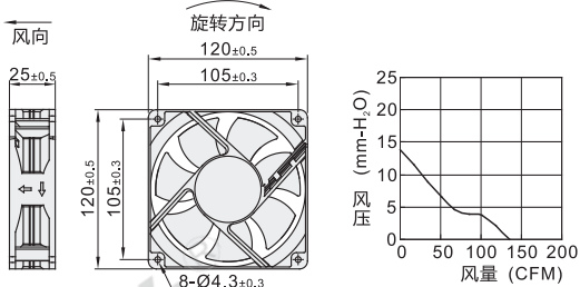
外形尺寸: 12038H
