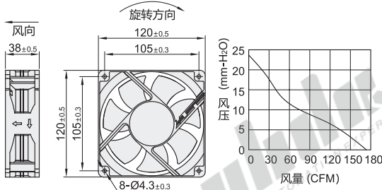
外形尺寸: 12038
