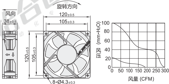
外形尺寸: 12038H
