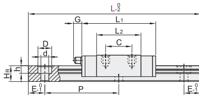
H(16)带注油嘴
