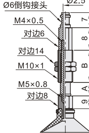
盘径Ø20~32
