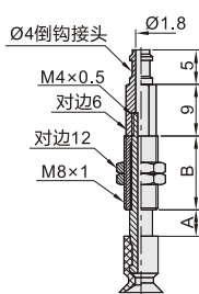
盘径Ø2~8
